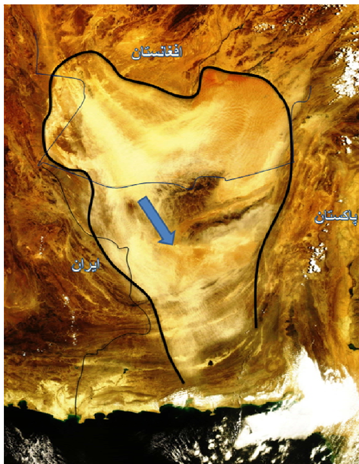
تصویر ۷ : طوفان عظیم ریگ و خاک در افغانستان (فراه، نیمروز، هلمند و قندهار)، ایران و پاکستان. تصویر از ناسا [۶]. اضافات از نگارنده. خط درشت حدود تقریبی طوفان، خط باریک سرحد بین افغانستان، ایران و پاکستان و تیر سمت وزش باد را از جانب شمال غرب به طرف جنوب شرق نشان می دهد.
