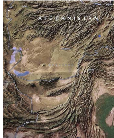
نقشه ۱ : حوزه فرو افتاده جنوبغرب افغانستان [۵]. نقشه ۲ : حوزه آبیگر هلمند با آبهای هامون هلمند. نقشه از نگارنده.
